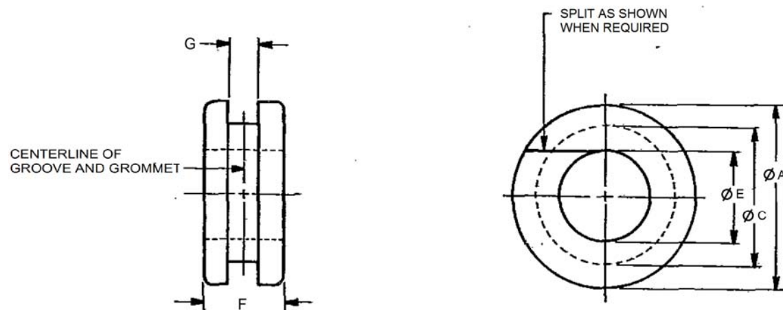
FIGURE 1. GROMMET.
